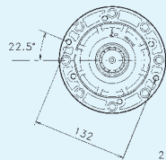
VISTA da A
