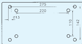
VISTA BASE POMPA
