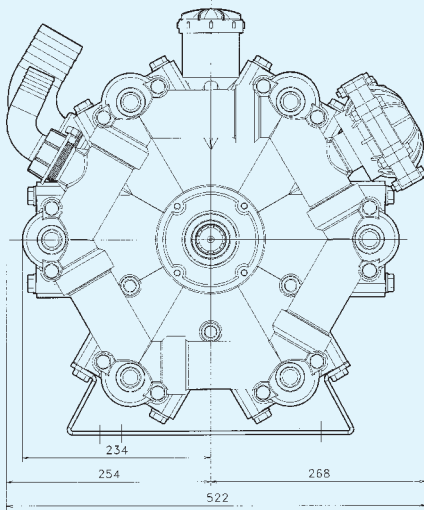
VISTA BASE POMPA
